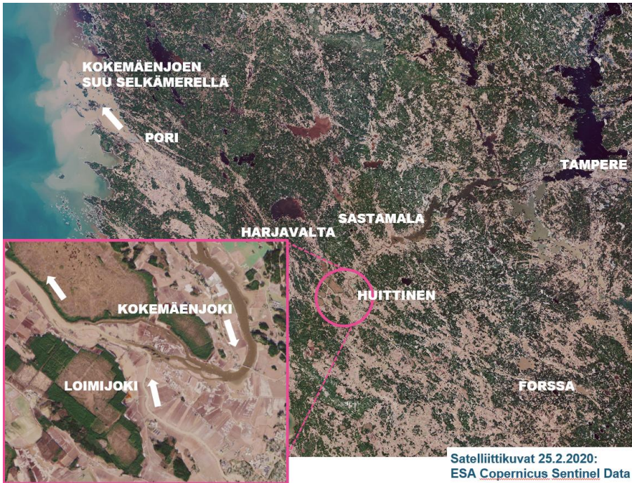
Kuva 2. Satelliittikuva Kokemäenjoen vesistöalueelta 25.2.2020 lauhan talven poikkeuksellisen runsaan sadejakson jälkeen. Tilanne havainnollistaa hyvin Loimijoen merkitystä Itämeren kuormittajana.
