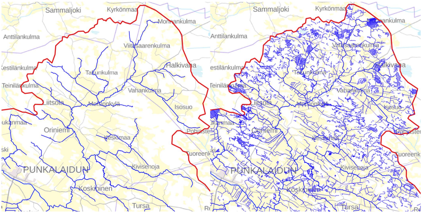
Kuva 3.1. Loimijoen vesistöalue on kauttaaltaan ojitettu ja vesi kulkee sateen jälkeen nopeasti eteenpäin. Kuvaparissa vasemmalla Punkalaitumen pohjoisosan luontaiset uomat ja oikealla nykyinen uomaverkosto.
