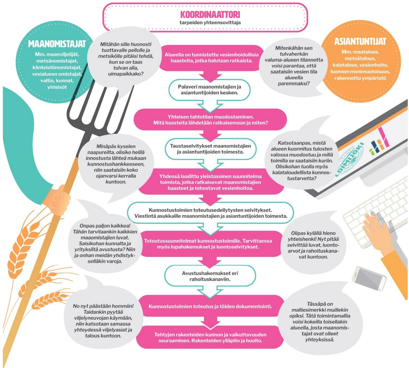
Kuva 3.2. Toimintamalli maanomistajien ja asiantuntijoiden yhteistyössä tehtävään kunnostussuunnitteluun.
